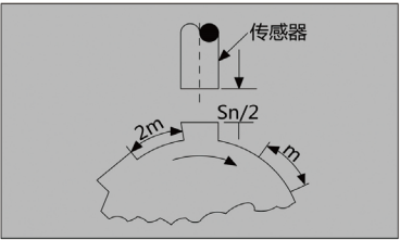
每秒钟， 开关动作的最大次数， 测量符合： EN 60947-5-2/IEC 947-5-2
