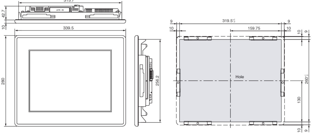
GC-A24W-C、 GC-A24W-RC GC-A24W-CW、 GC-A24W-RCW
