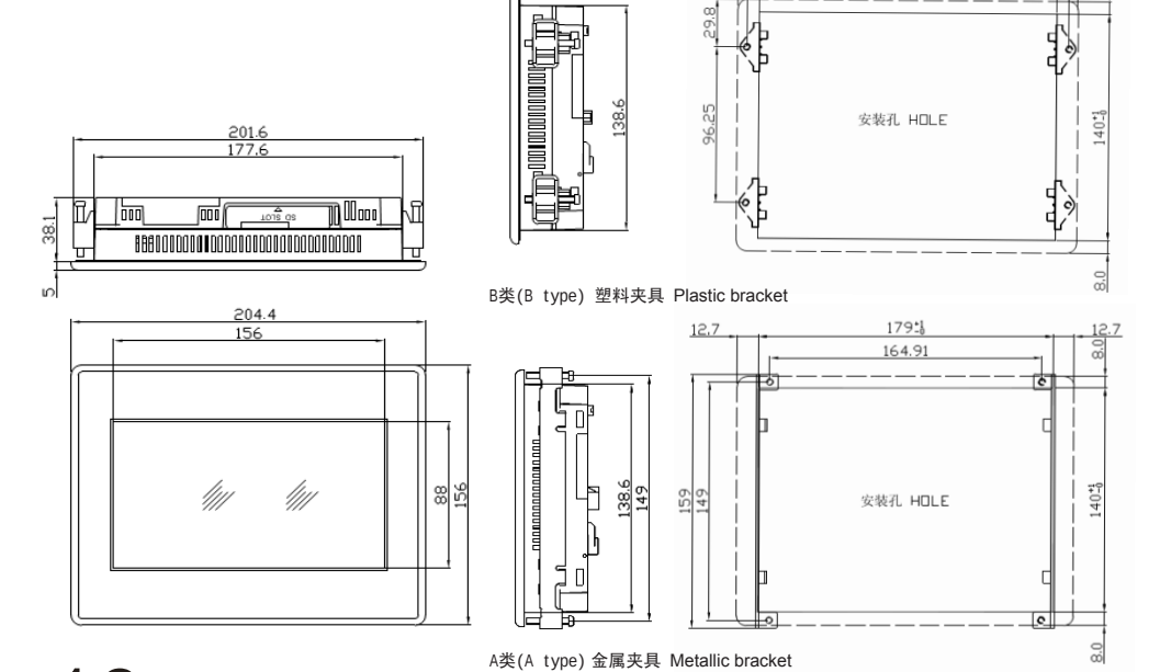
A类(A type) 金属夹具 Metallic bracket
