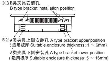
GC-A26W-C、 GC-A26W-RC GC-A26W-CW、 GC-A26W-RCW
