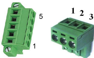
5 连端子插头
