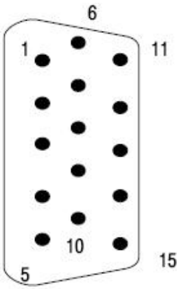
15 脚孔型 D 型插座
