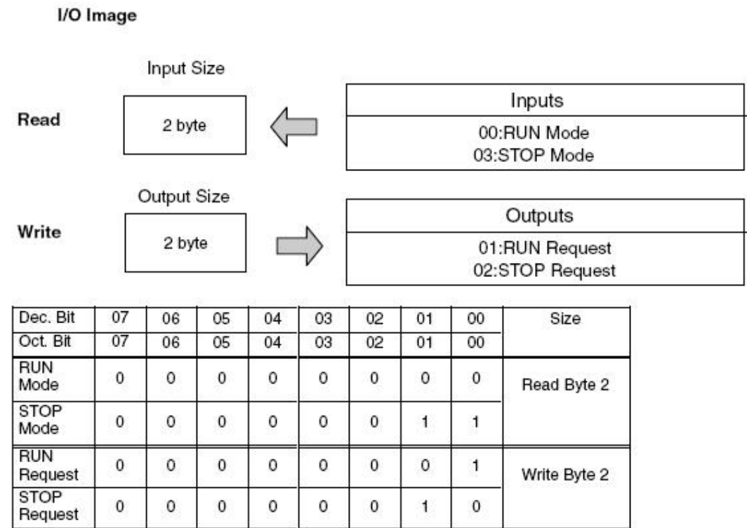
PLC 模式映射表
