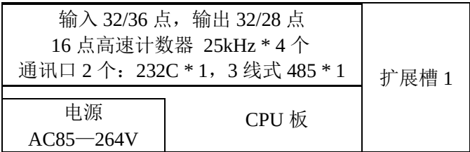
SN64DR(D)-A3/B3 功能结构图
