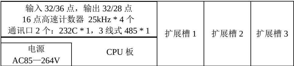
SN64DR(D)-A3/B3 功能结构图
