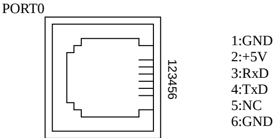
(2) SN 与手持编程器 S-200HP 接线图
