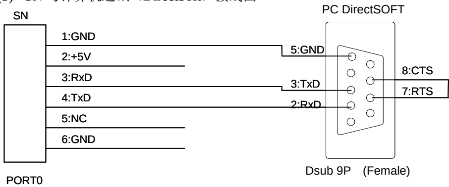
(3) SN 与计算机通讯 (DirectSoft) 接线图
