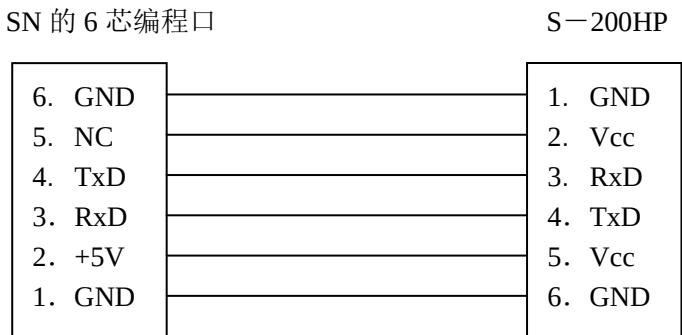
(2) SN 与手持编程器 S-200HP 接线图
