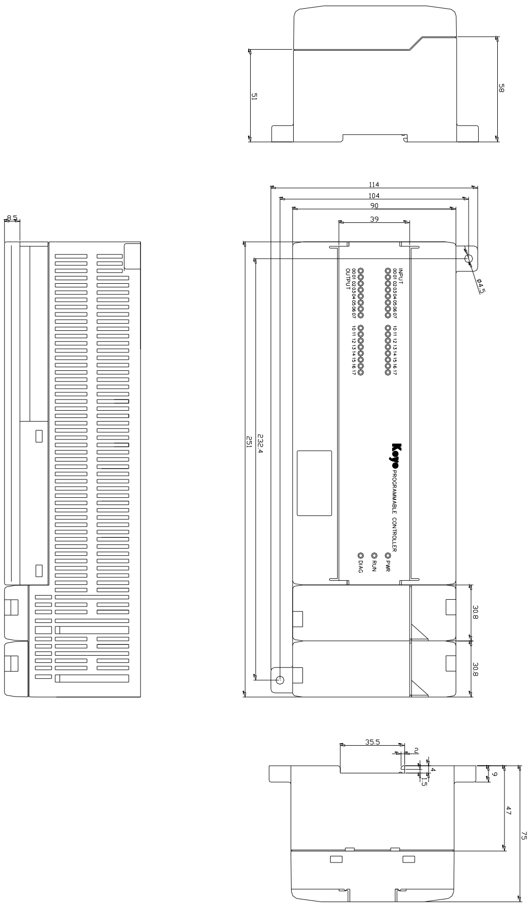
② SN32DR-A2/B2(SN32DD-A2/B2)外形和安装尺寸图：
