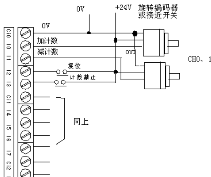
C) A/B 相输入接线例
