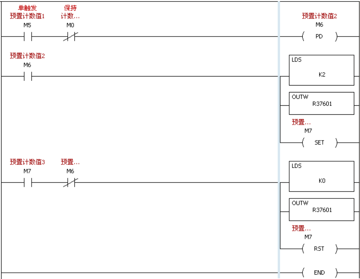
4) 预置计数值功能实现程序段
