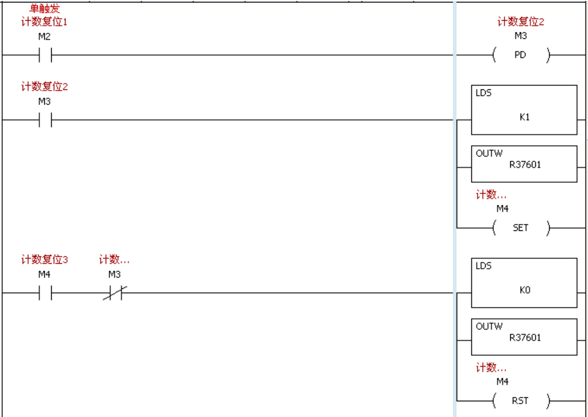
4) 预置计数值功能实现程序段
