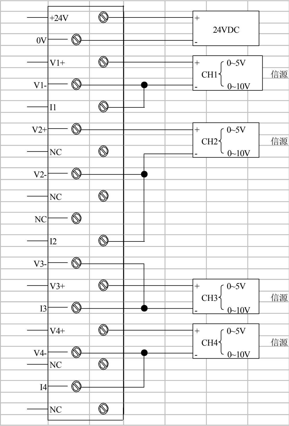
4-5-1 电压输入方式时的接法
