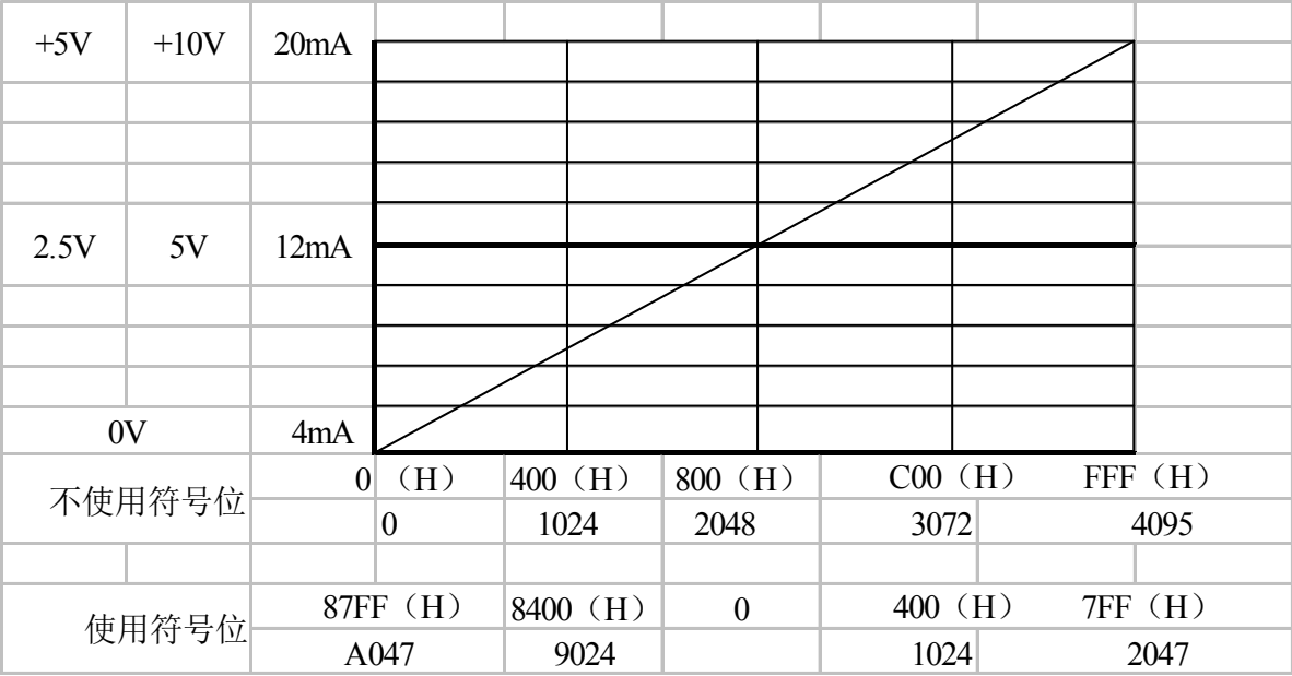
7-3、数模转换图
