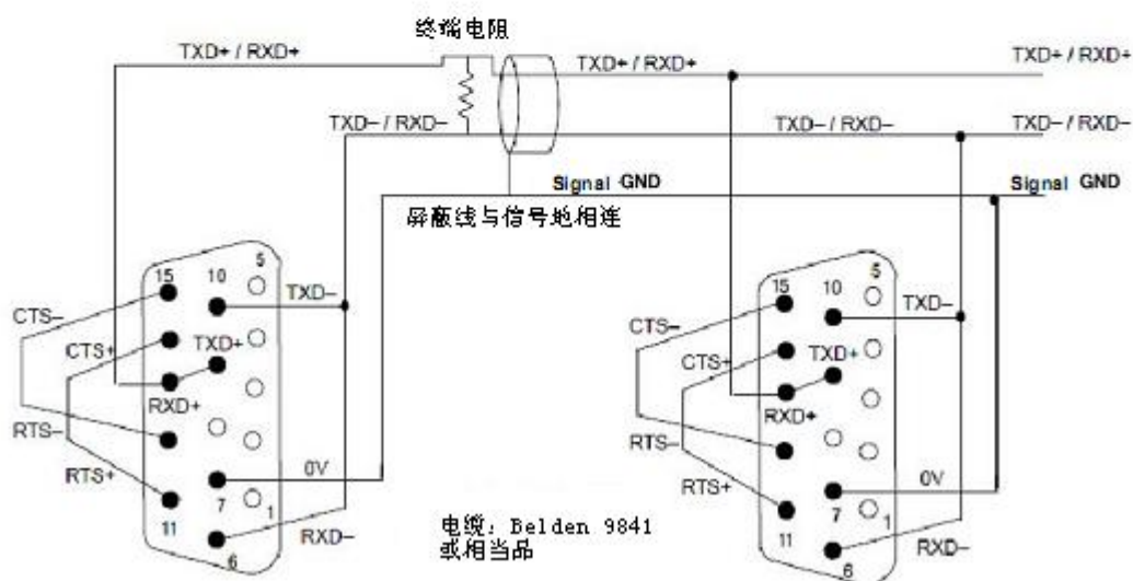
RS-485 网络
