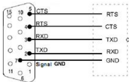
RS-232C 网络
