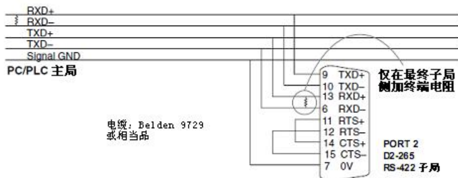
RS-422 网络
