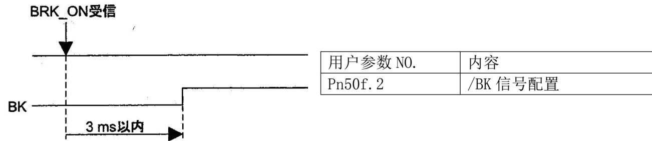
制动信号输出时序
