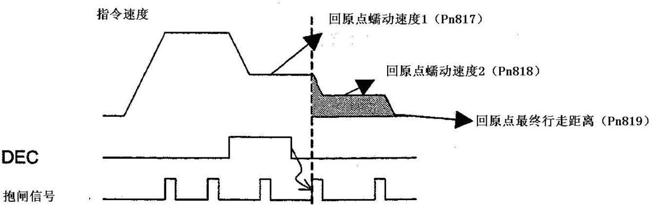
回原点时序图
