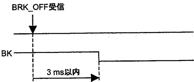
制动解除信号的时序
